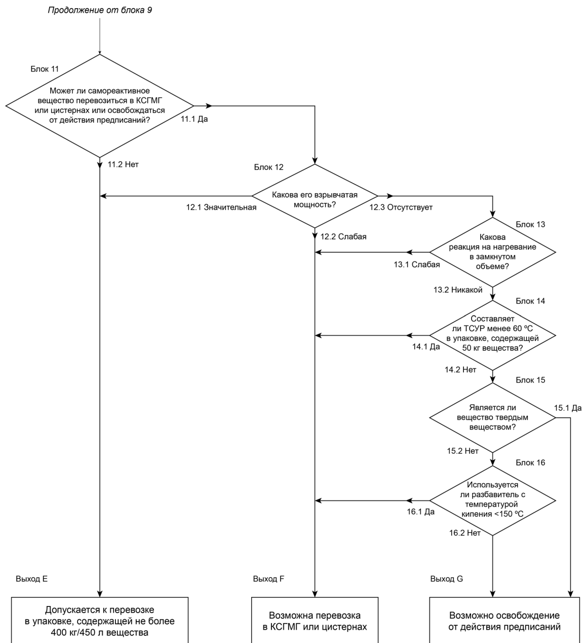
Рисунок Б.7, лист 2
