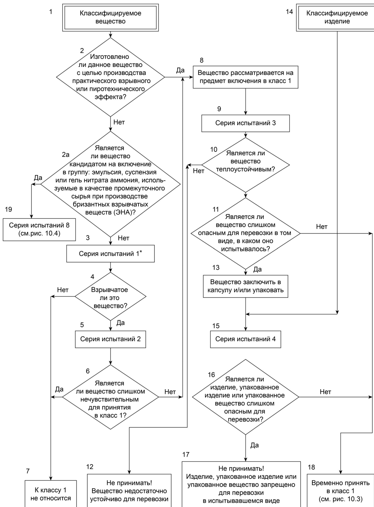
Рисунок Б.8 — Схема процедуры временного принятия вещества или изделия в класс 1
