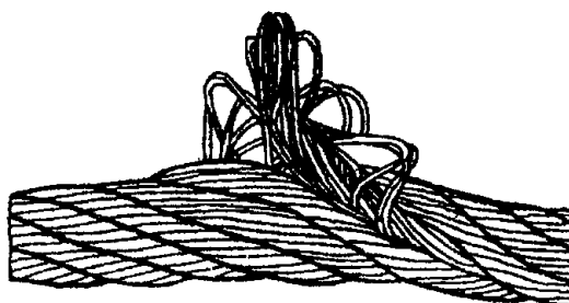
Рисунок 10. Корзинообразная деформация
